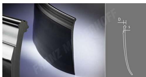
afsluitrubber BR33P
