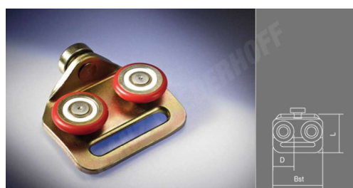
dubbele runner gelagerd (enkelzijdig + ) voor EDSCHA rail gleuf 50mm
