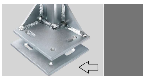
tegenplaat voor hoekpaal
